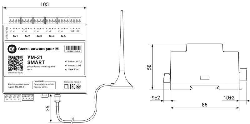
Рисунок 1. Габаритные размеры устройства
